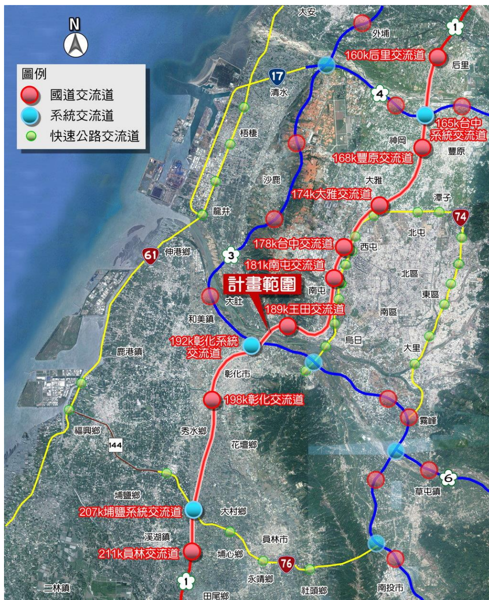
國道 1 號臺中至彰化路段興建高架道路之先期評估範圍示意圖
